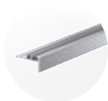
Profilé Incizo / Profilé de base en aluminium Incizo pour escaliers QSVINCP(-) / NEVINCPBASE1 2 000 x 45 x 8 mm / 2 000 x 33 x 17 mm
