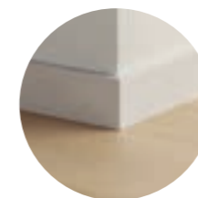
Streichbare Standard-Sockelleiste QSSKPAINT 2400 × 12 × 58 mm
