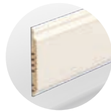
Streichbare Sockelleiste Modell Ogee QSISKROGEE 2400 x 16 x 160 mm
